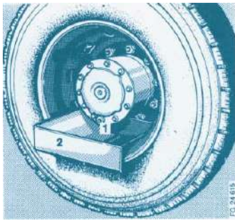
Бортовой редуктор HL7, HD7
