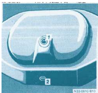
Приводной передний мост AL7 1. заливная пробка 2. сливная пробка
